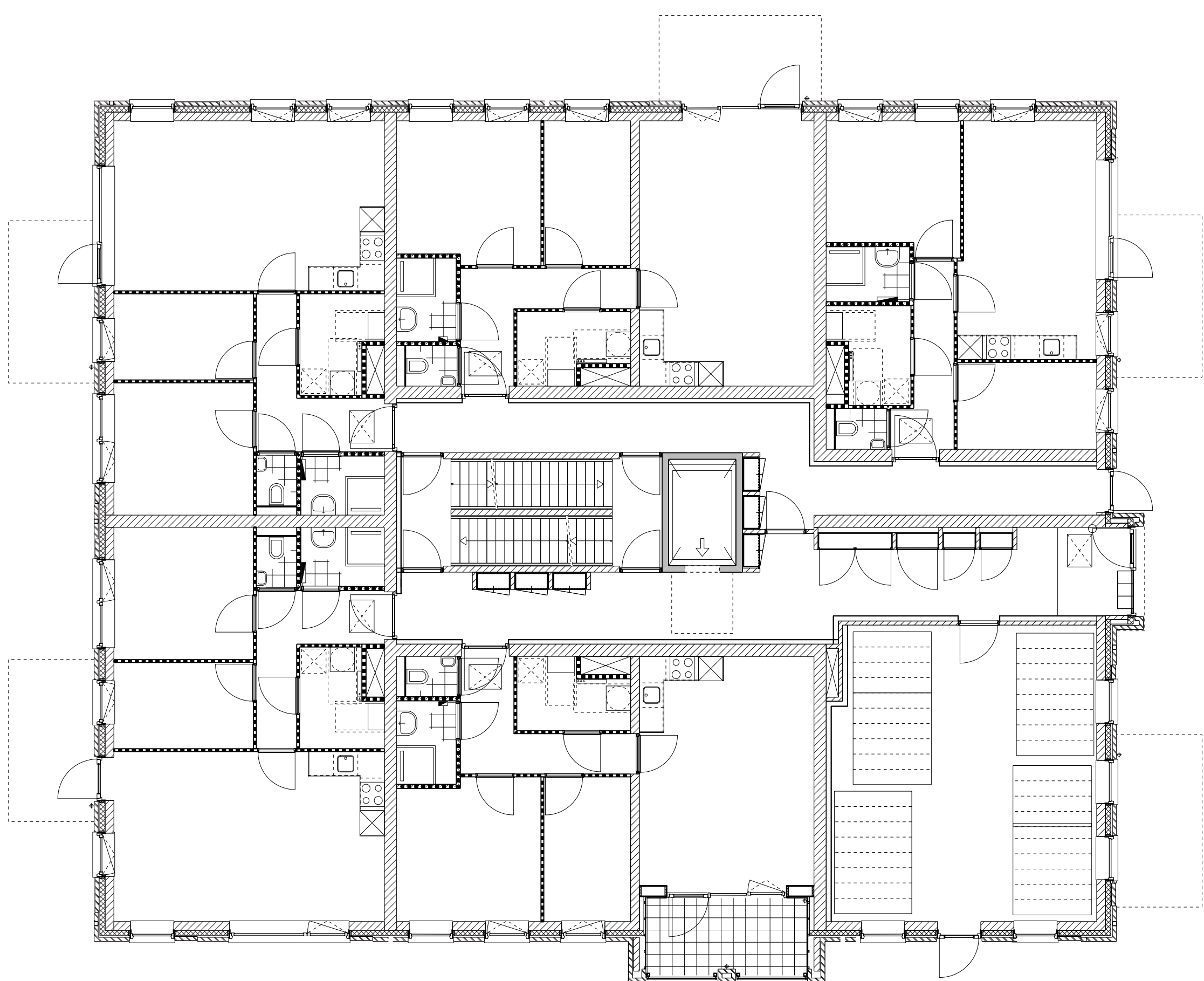
BEGANE GROND
