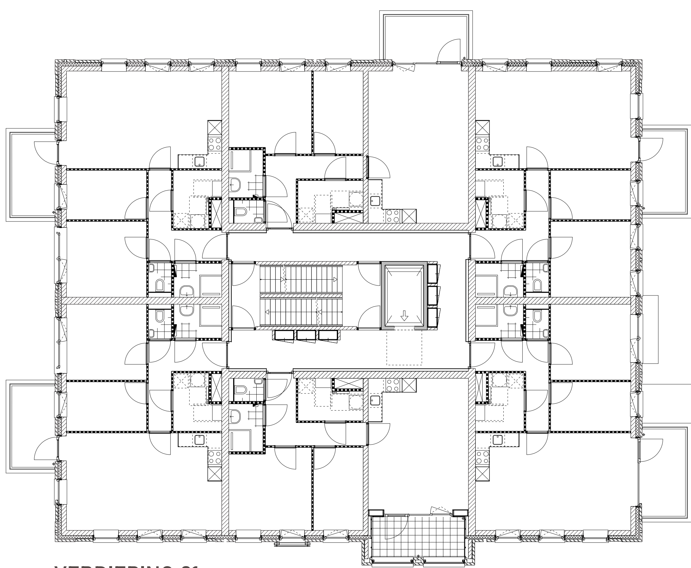
VERDIEPING 01
