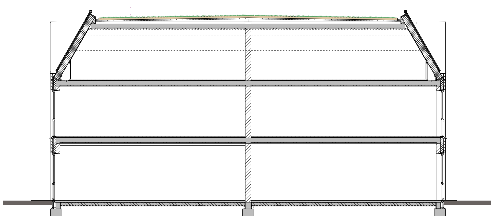
DOORSNEDE
