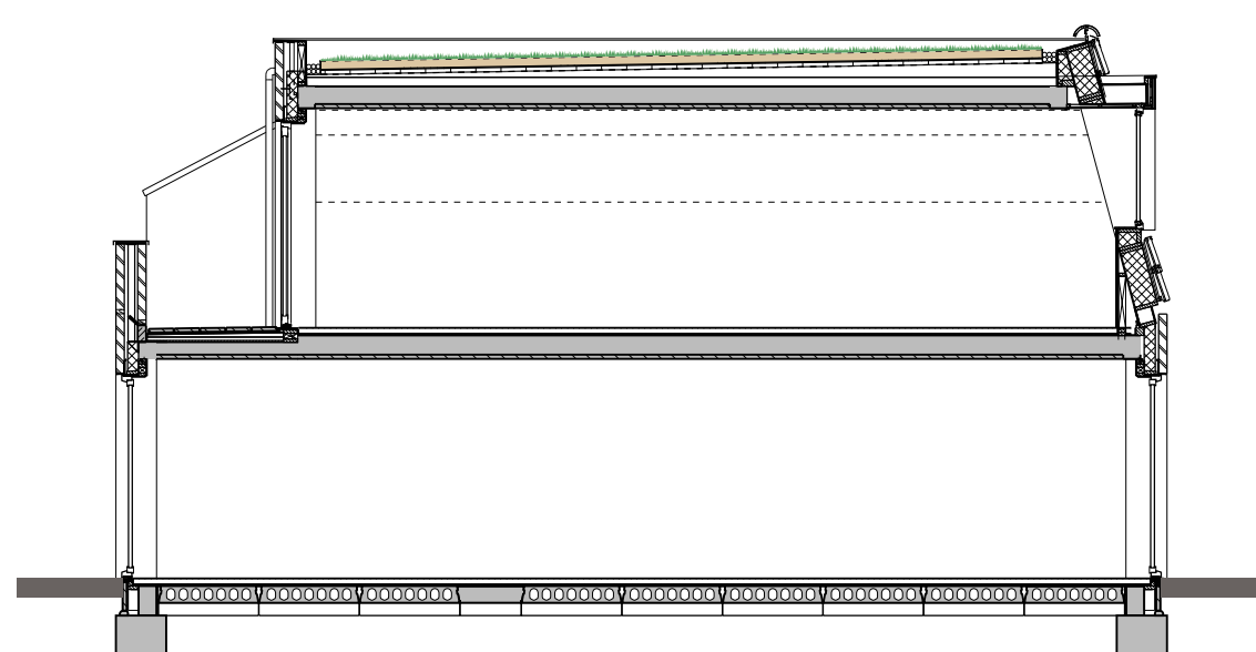
DOORSNEDE
