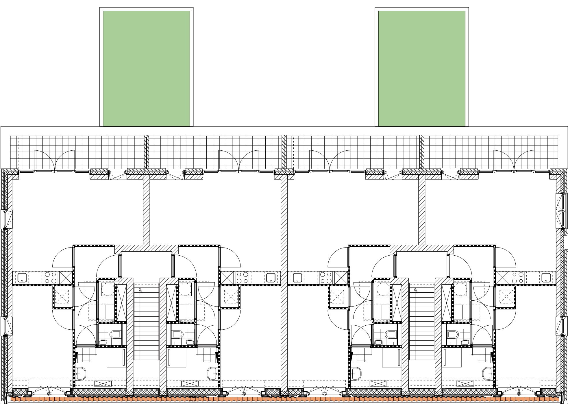
VERDIEPING 01
